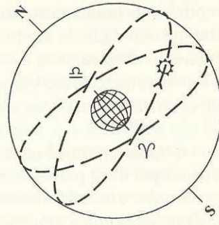
FIGURA 15 - A elíptica e os equinócios
