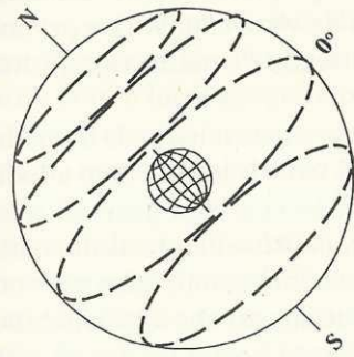
FIGURA 14 - Os pólos e o equador celestes
